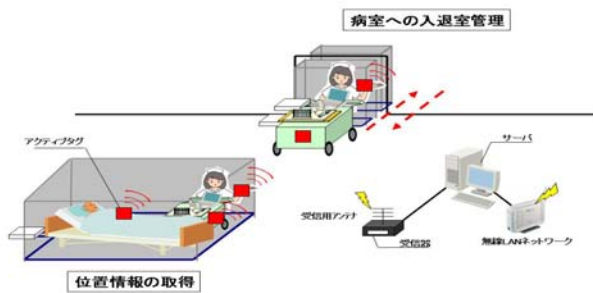
図1 トリガー磁界方式アクティブタグ
